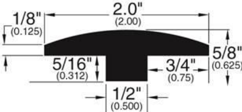
T-Mold (002)
